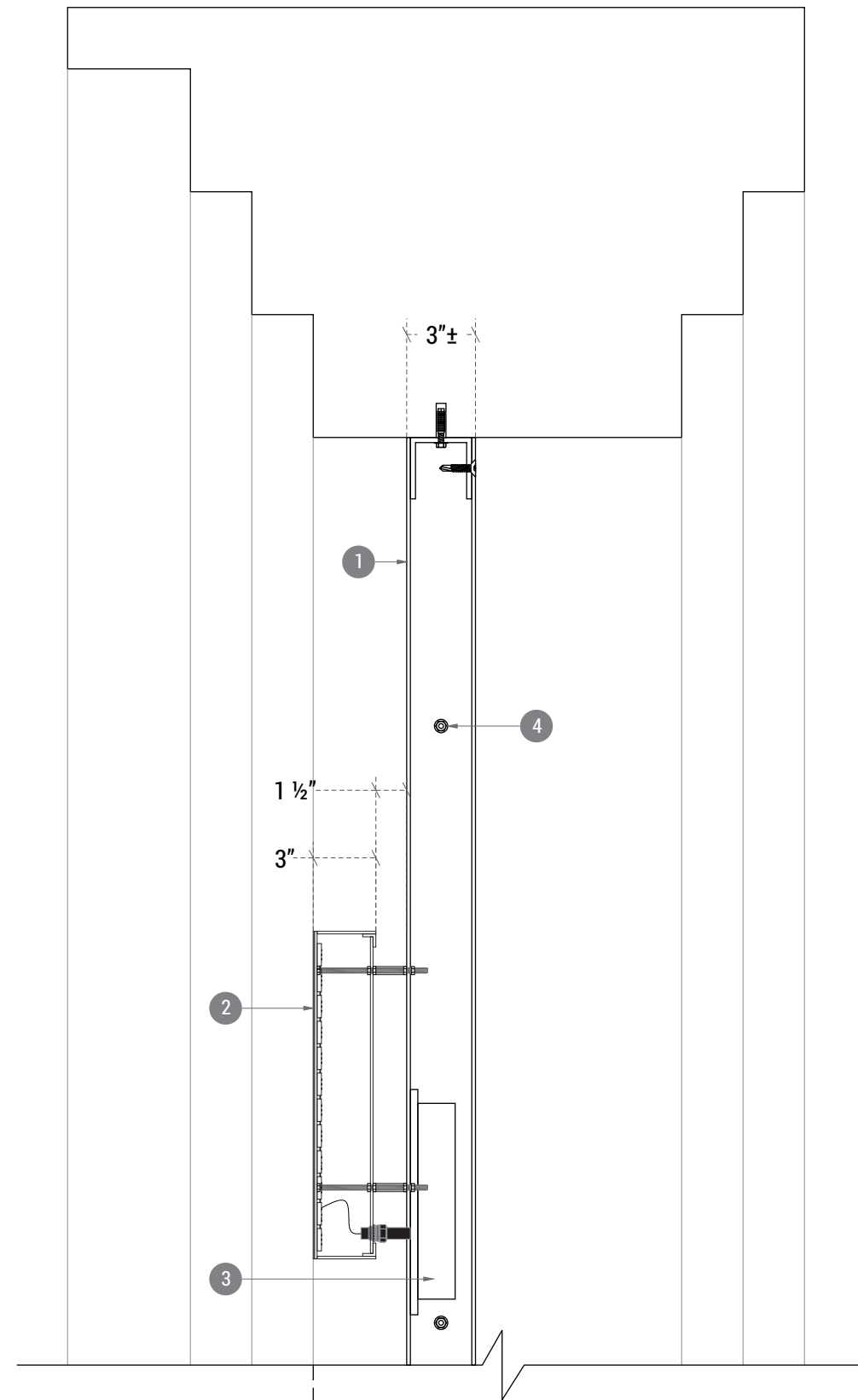
A SECTION SCALE: 1 1/2"=1'-0"
